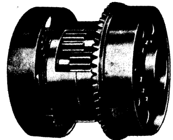
Ausgleichgetriebe
